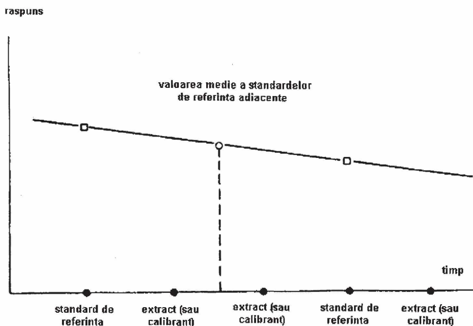
Figura 3*): Compensarea aglomerării în răspunsul aflatoxinei B prin injectarea standardului de referință (3.13.3) la intervale regulate de timp
