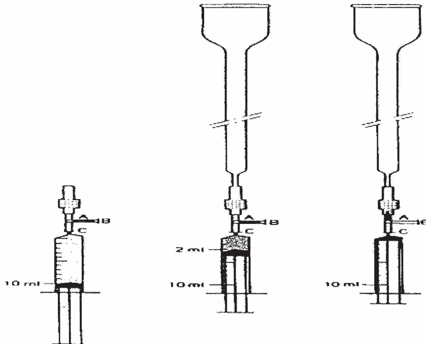
Figura 1*): Ansamblul coloană-cartuș
